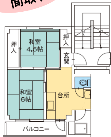
間取り
